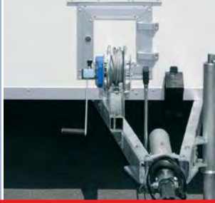
Seilzugwinde
